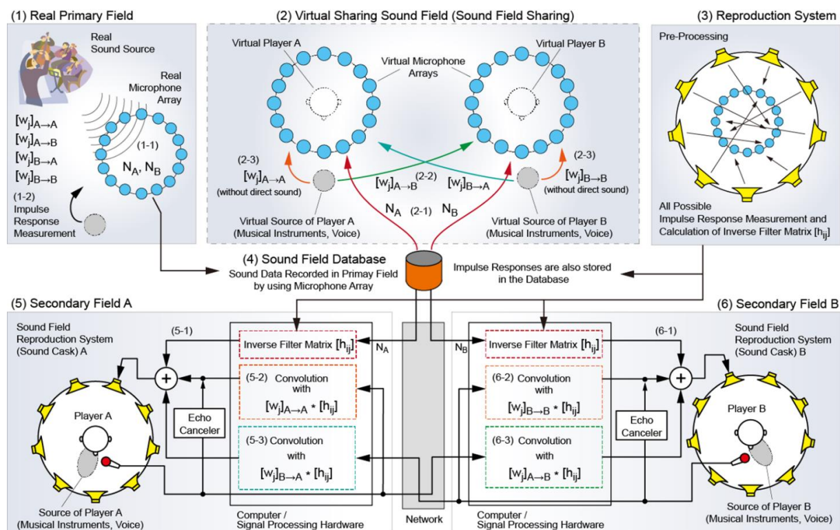
図5 聴空間共有システムの全体構成
